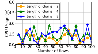
(d) CPU usage of eMPTCP.
